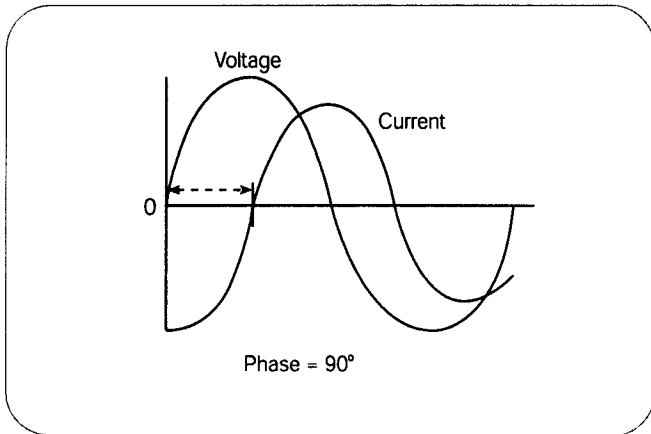
► Figure 12. Phase shift.
